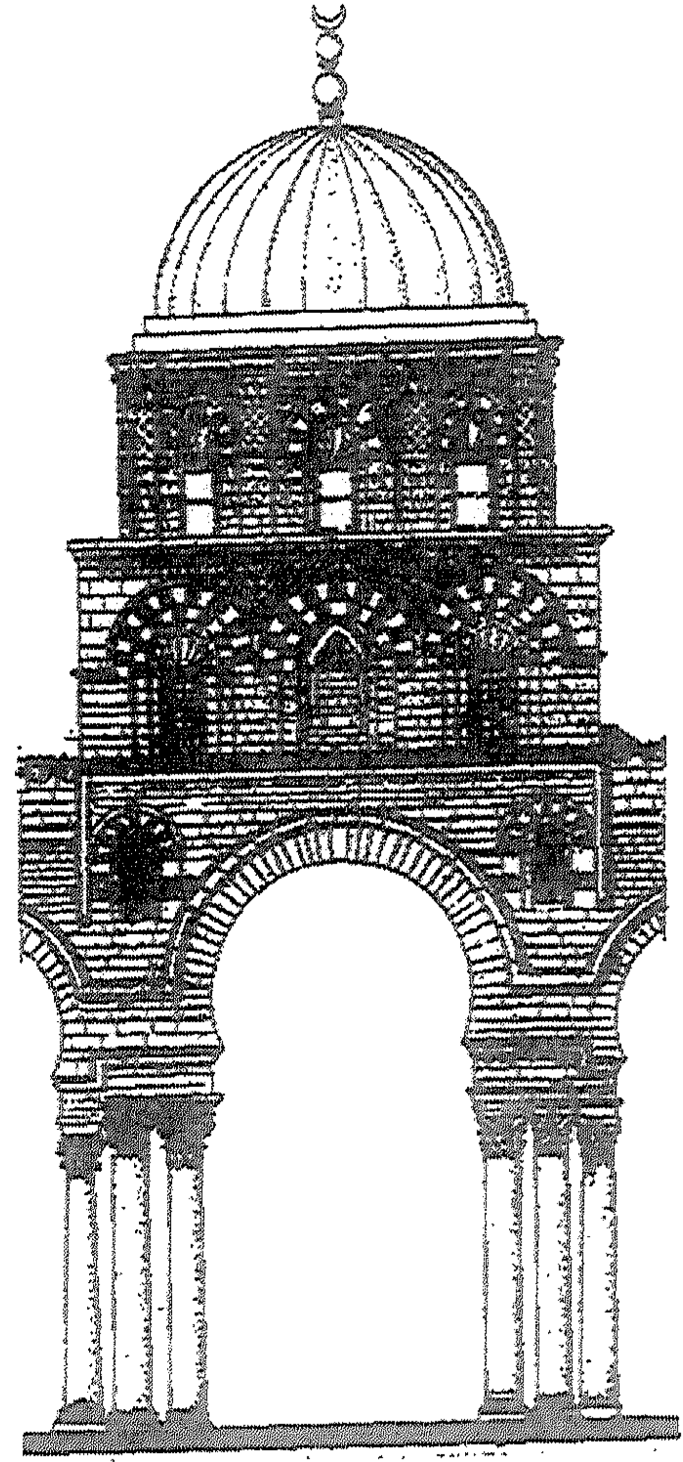
(شكل رقم ٧٤) واجهة قبة البهو بجامع الزيتونة عن د/ الدولاتلى.
